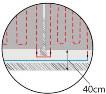
FLEXIRO Wandheizung, Detailausschnitt Verbindung der Elemente
