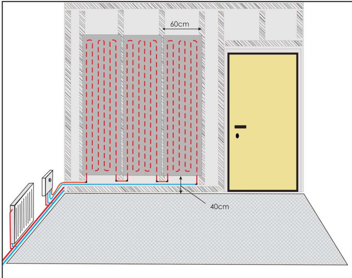
FLEXIRO Wandheizung, drei Wandelemente
