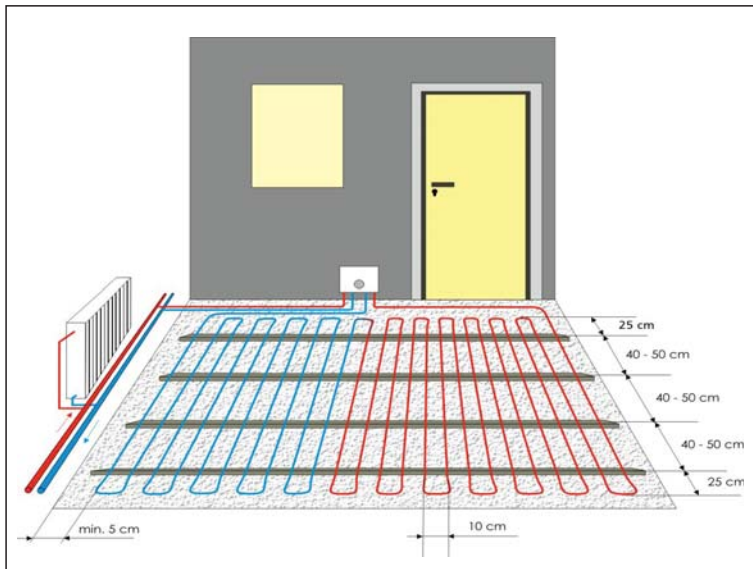
FLEXIRO Dünnbett Fußbodenheizung, Verlegeform: mäanderförmig
