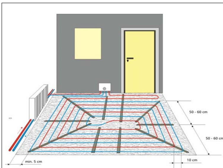
FLEXIRO Dünnbett Fußbodenheizung, Verlegeform: spiralförmig
